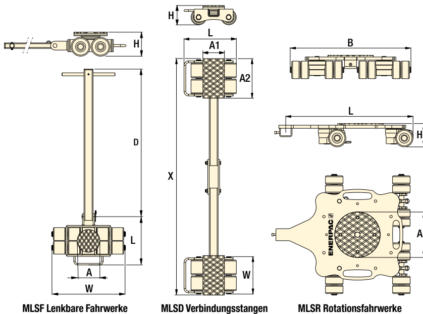
MLSF Lenkbare Fahrwerke
